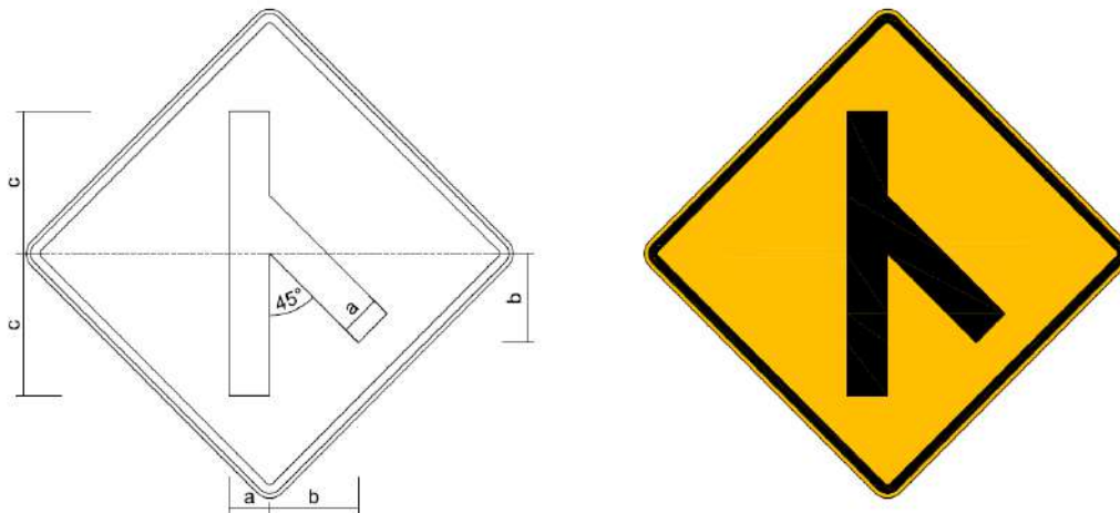
Figura A.76 – Placa A-13b – Confluência à direita
