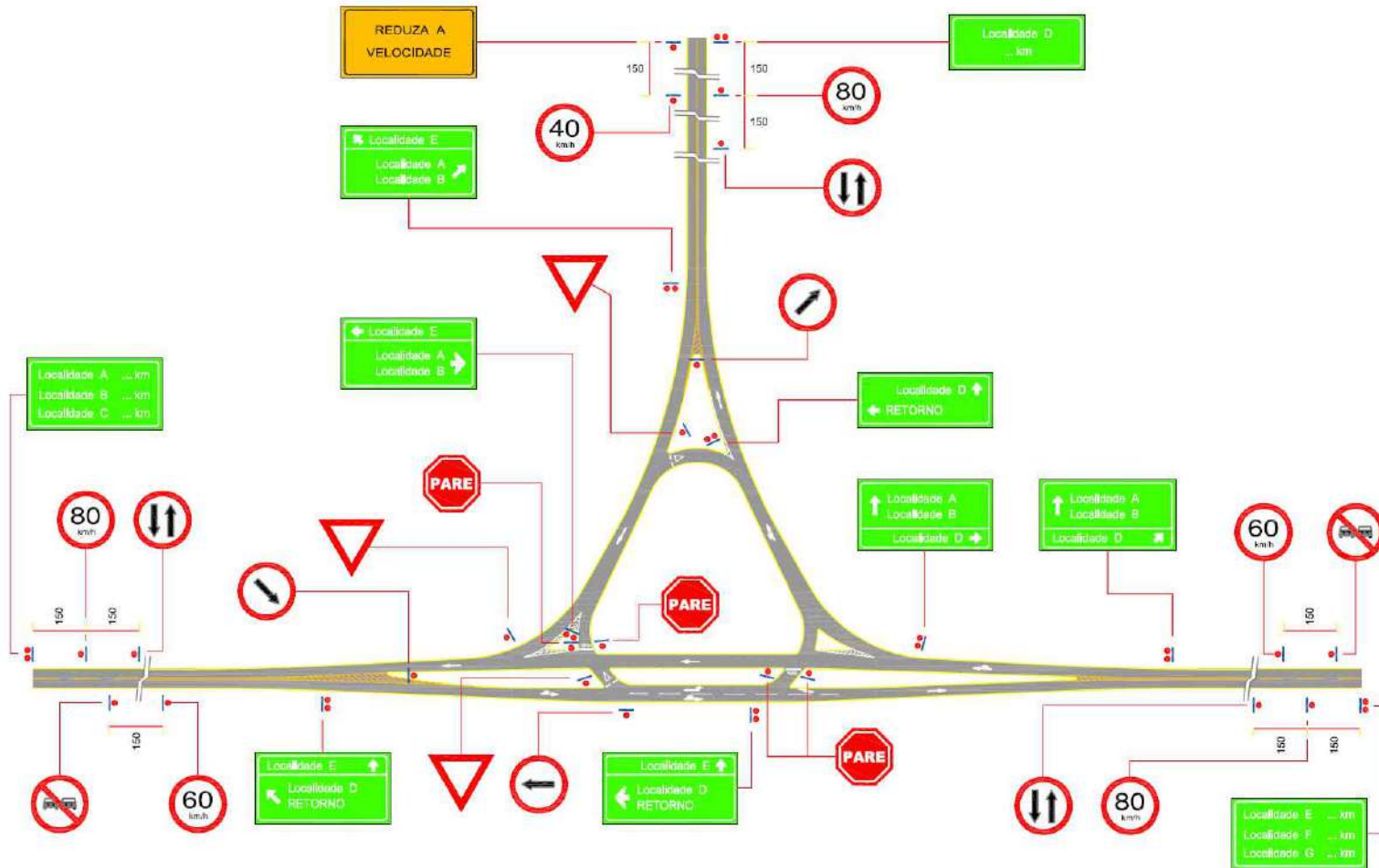
Figura 267 – Interseção em nível
