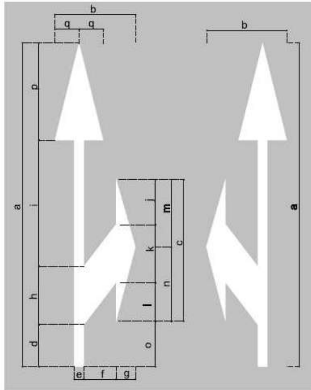
Figura 249 – Setas “siga em frente ou vire à direita” e “siga em frente ou vire à esquerda”
