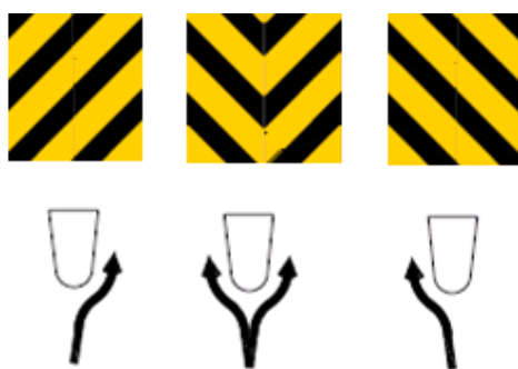
Figura 217 – Marcadores de obstáculos
