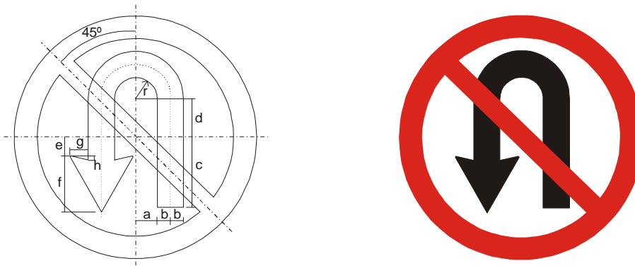
Figura A.8 – Placa R-5a – Proibido retornar à esquerda
