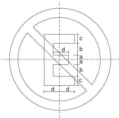
Figura A.10 – Placa R-6a – Proibido estacionar
