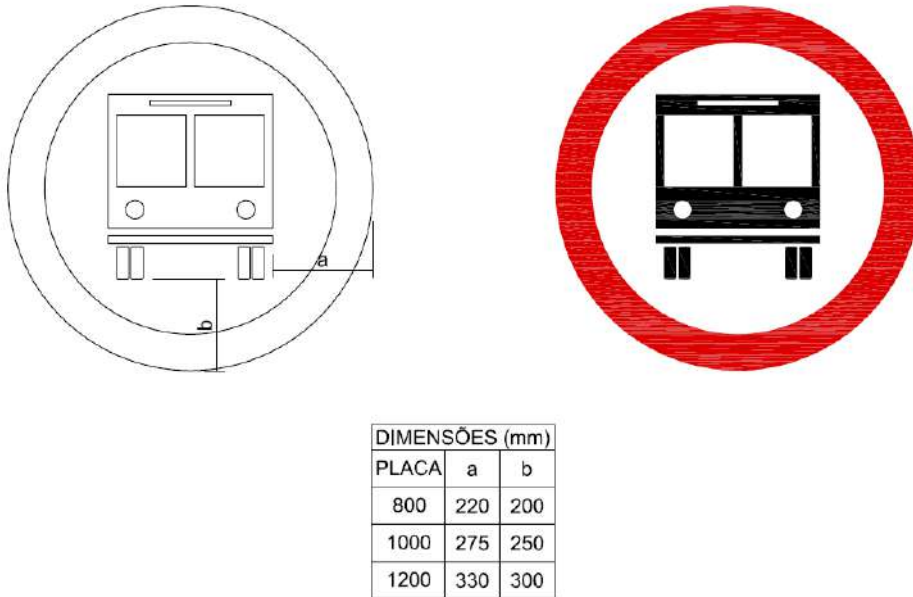
Figura A.43 – Placa R-32 – Circulação exclusiva de ônibus
