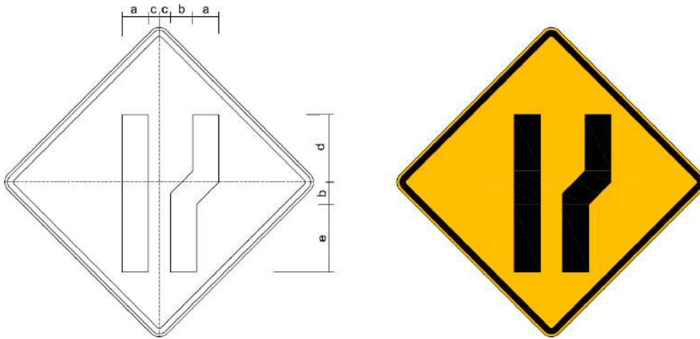
Figura A.89 – Placa A-21e – Alargamento de pista à direita
