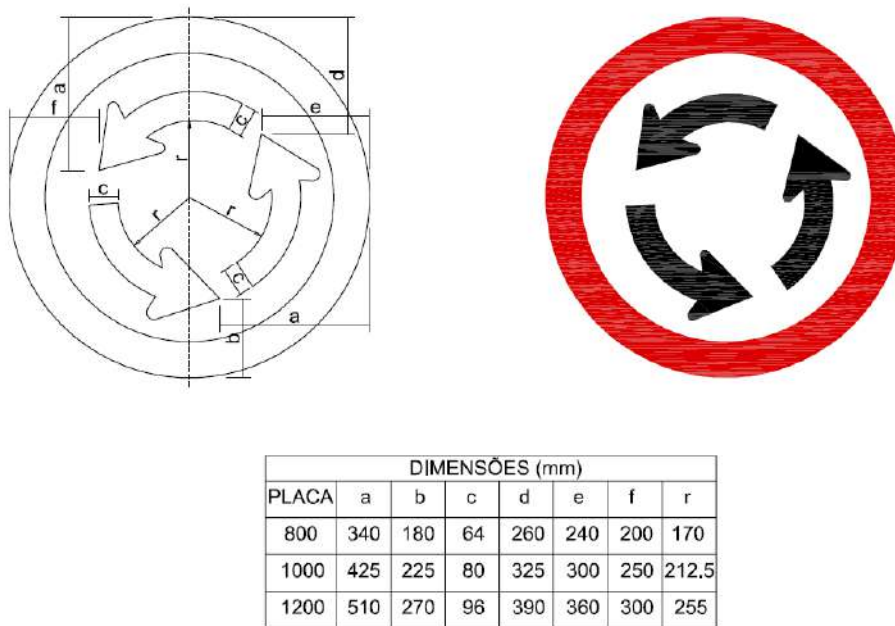
Figura A.44 – Placa R-33 – Sentido de circulação na rotatória
