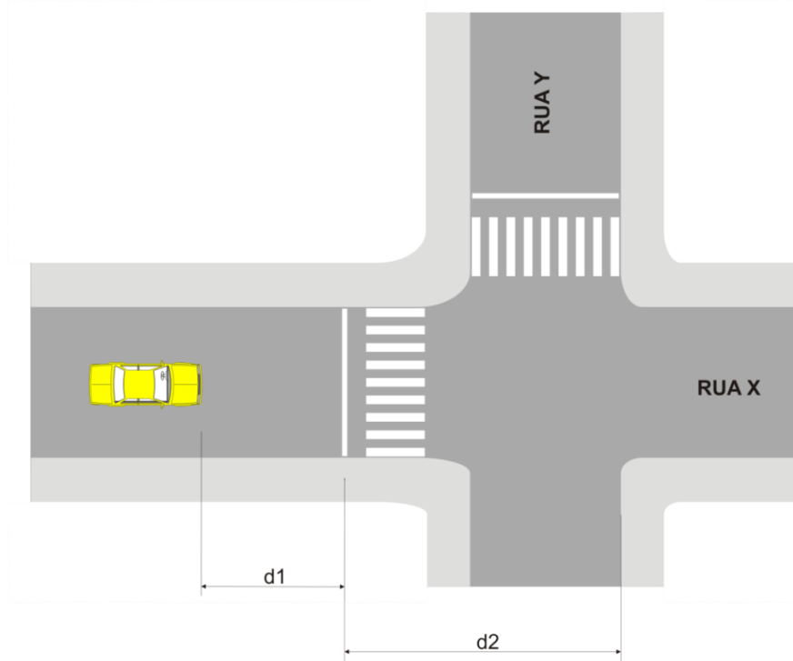
Figura 6.6: Distâncias percorridas pelo veículo junto à aproximação
