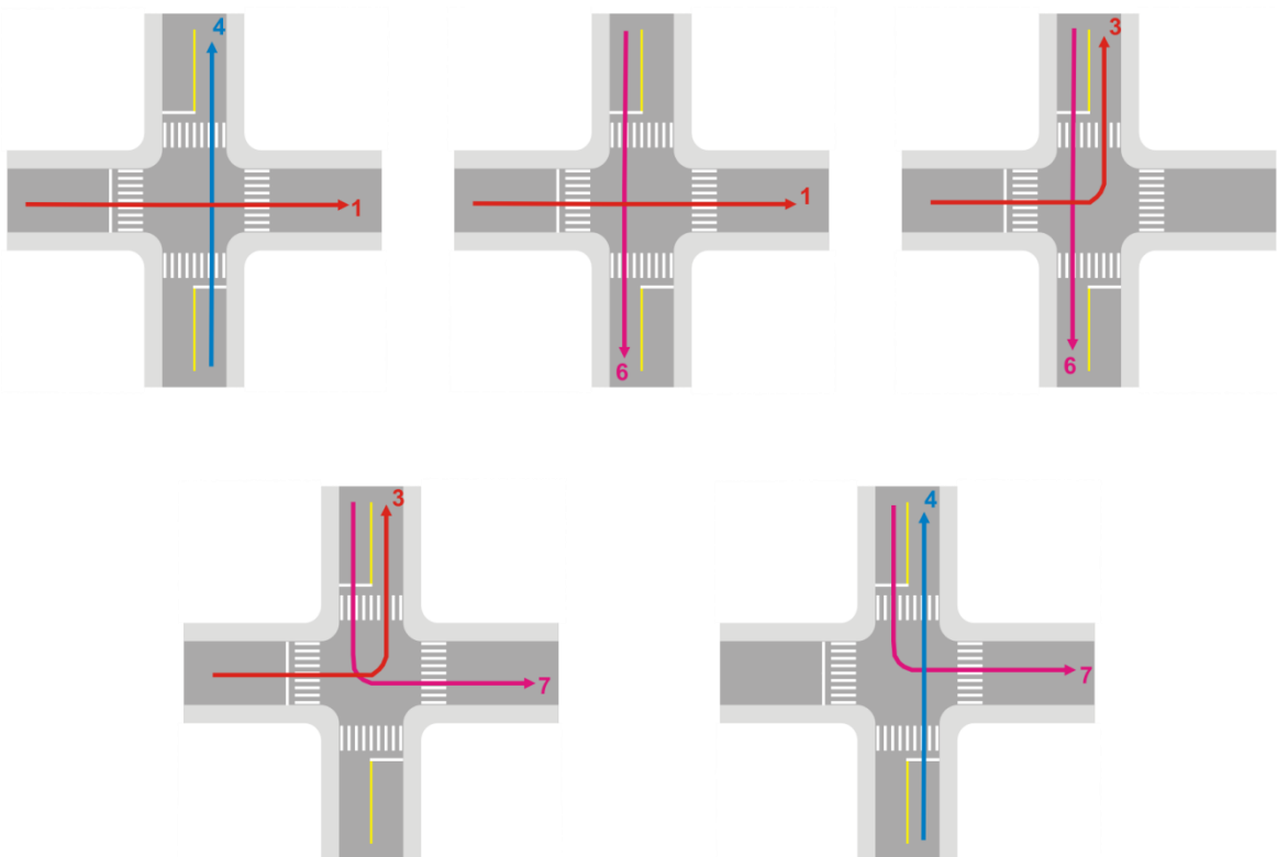
Figura 4.5: Movimentos interceptantes
